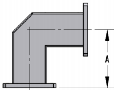
E-Plane
